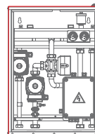
Kit DMC (disgiuntore miscelato con valvola motorizzata)
