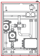
Kit DMT (disgiuntore miscelato con valvola termostatica manuale)
